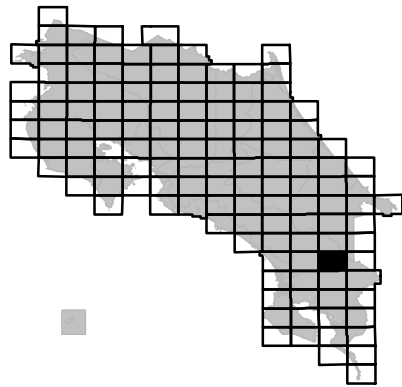
Mapa de ubicación de la hoja Cabagra
