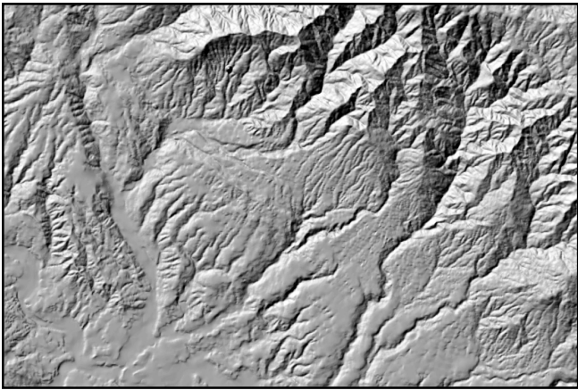
Modelo digital de relieve, hoja Cabagra; Relieve sombreado SRTM Level 1 (3-arc sec)
